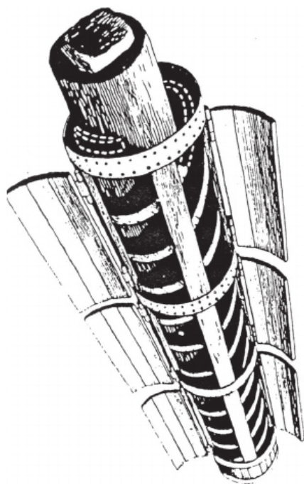
Figura 1.1: Coclea, ricostruzione grafica da reperto secondo un esemplare rinvenuto nelle miniere di Sotiel in Spagna
