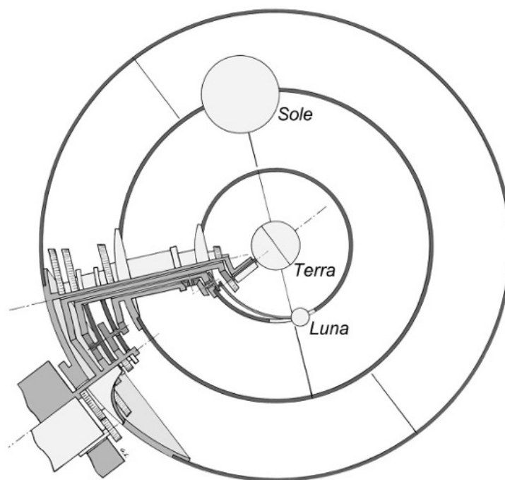
Figura 1.2: Ipotetica ricostruzione del planetario di Archimede; da brunelleschi.imss.fi.it
